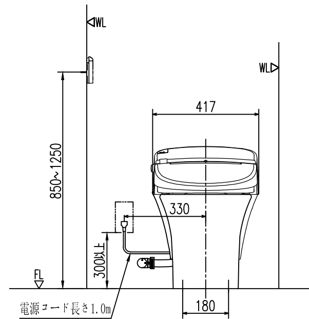
リモコン正面図
