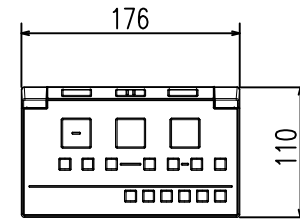
リモコン正面図
